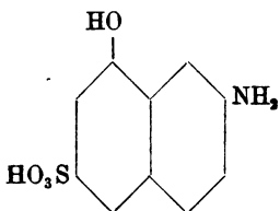
Aminonaphtolsulfosäure G.
